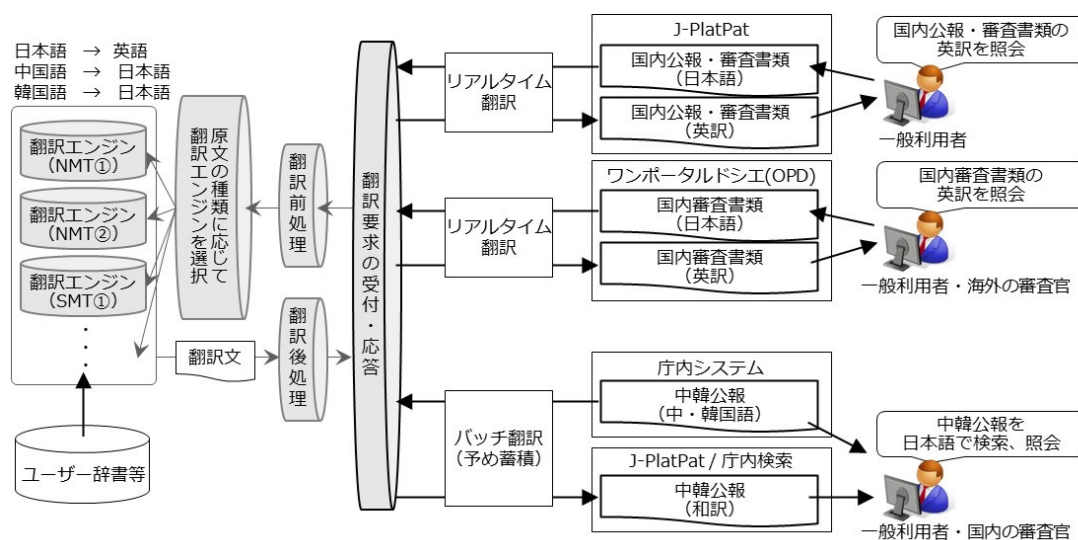
図１ 機械翻訳プラットフォームの概要
